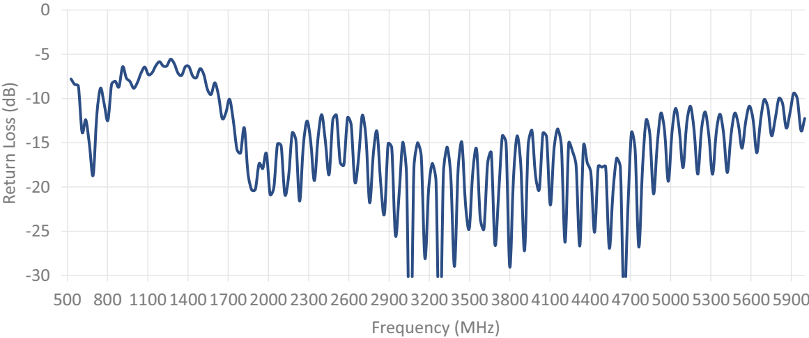
Cable 2: 5GNR
