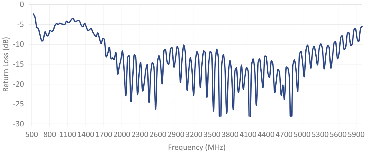
Cable 1: 5GNR
